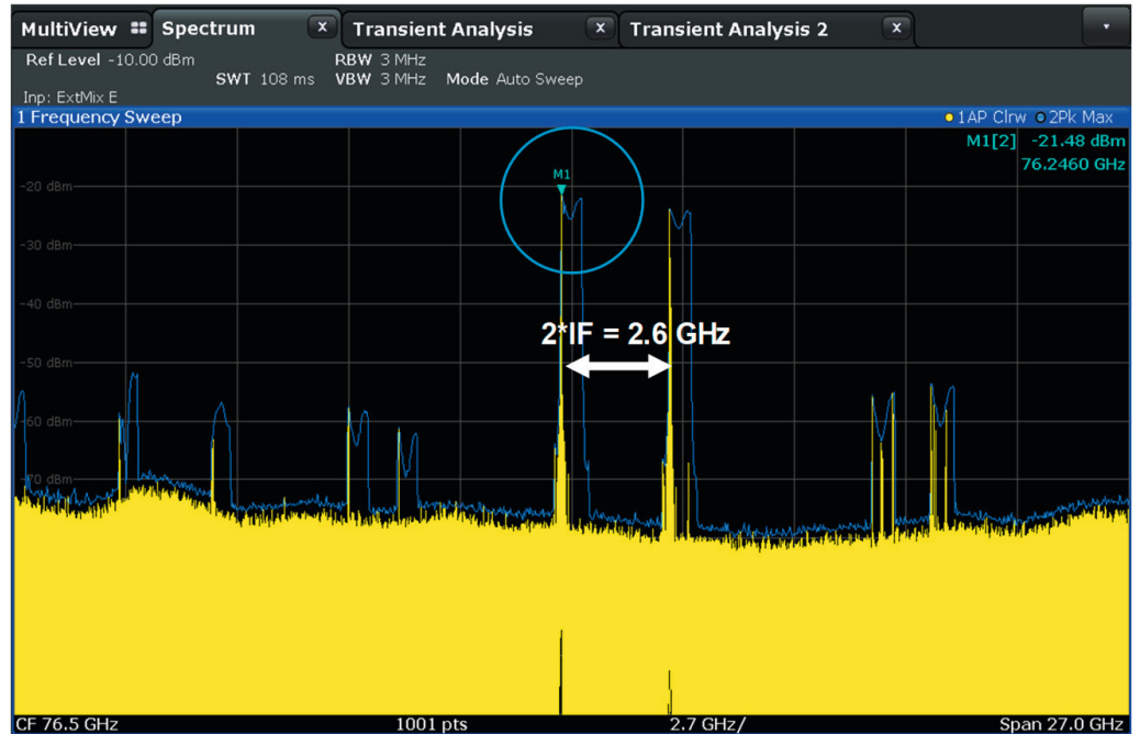
図3：R&S®FSW43に接続されたR&S®FS-Z90外付けハーモニック・ミキサで測定した60 GHz ~ 90 GHzのスペクトラム。76 GHzの希望信号は500 MHz幅です。最も近い画像は、スペクトラム・アナライザの中間周波数の2倍になります。他の不要な混変調信号およびそのイメージも存在します。
