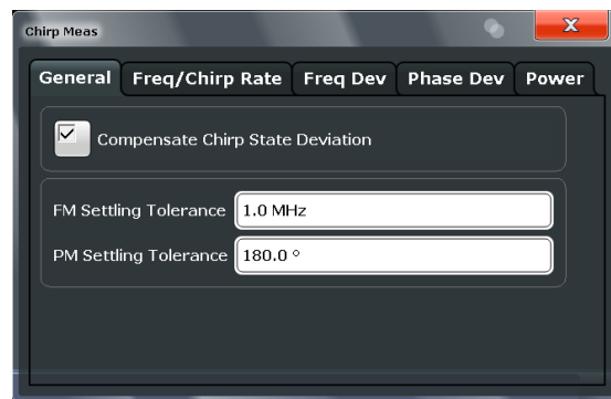
図13：デフォルトでは、測定されたチャープレートがチャープ直線性測定を実行するために使用され、平均チャープ状態からのずれが補償されます。
