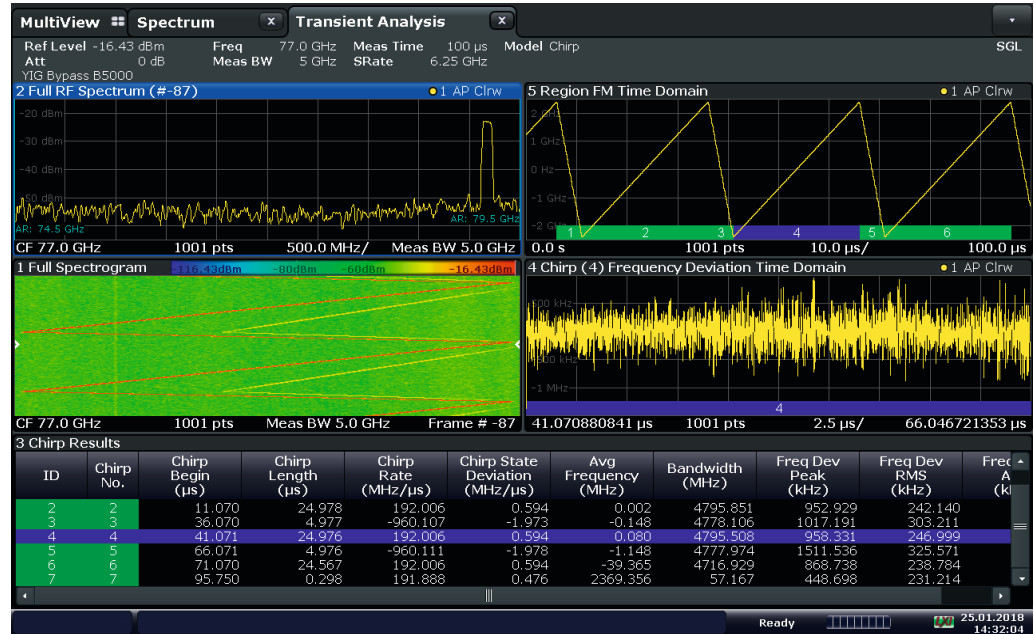
図10：R&S®FSW-K60C トランジェント測定アプリケーション
