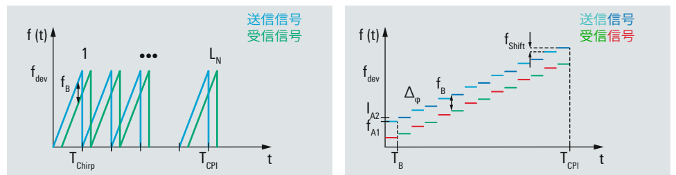
図8：周波数変調連続波 (FMCW) チャープ波形 (左) 対 多周波数シフトキーイング (MFSK) 波形 (右)
