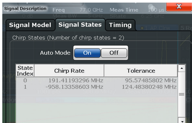
図11：R&S®FSW-K60Cアプリケーションの信号記述表、チャープ自動検出 (自動モード：オン)
