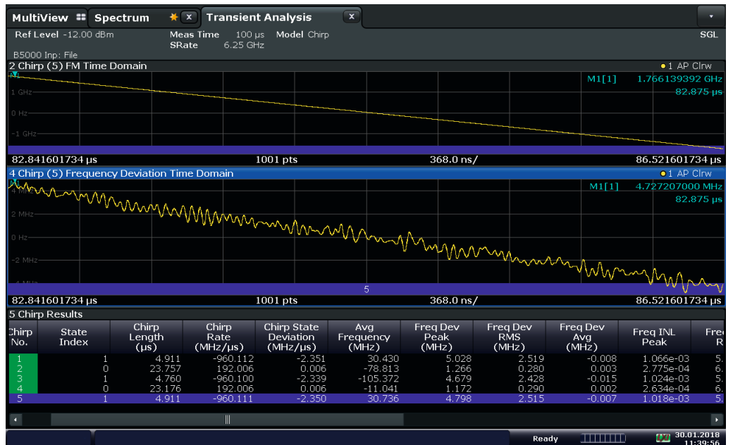
図15：測定された平均チャープレート（ベストフィット）の代わりに、信号記述テーブルの公称チャープレートを基準として計算された周波数偏差
