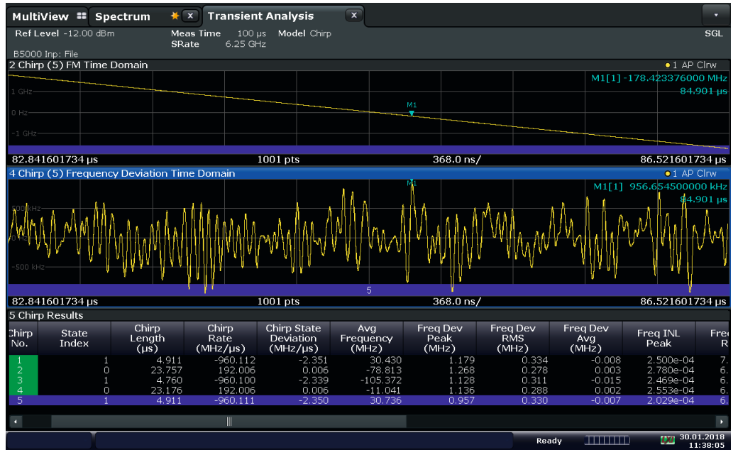
図14：ベストフィット測定手法による直線性測定の例。チャープ5に焦点を当てる；FM時間領域および周波数偏移時間領域パラメータ
